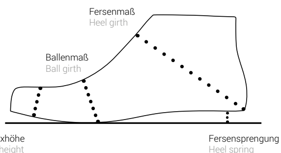
Umfangmaße vom Bruttoleisten Circumferences (gross shoe last)
